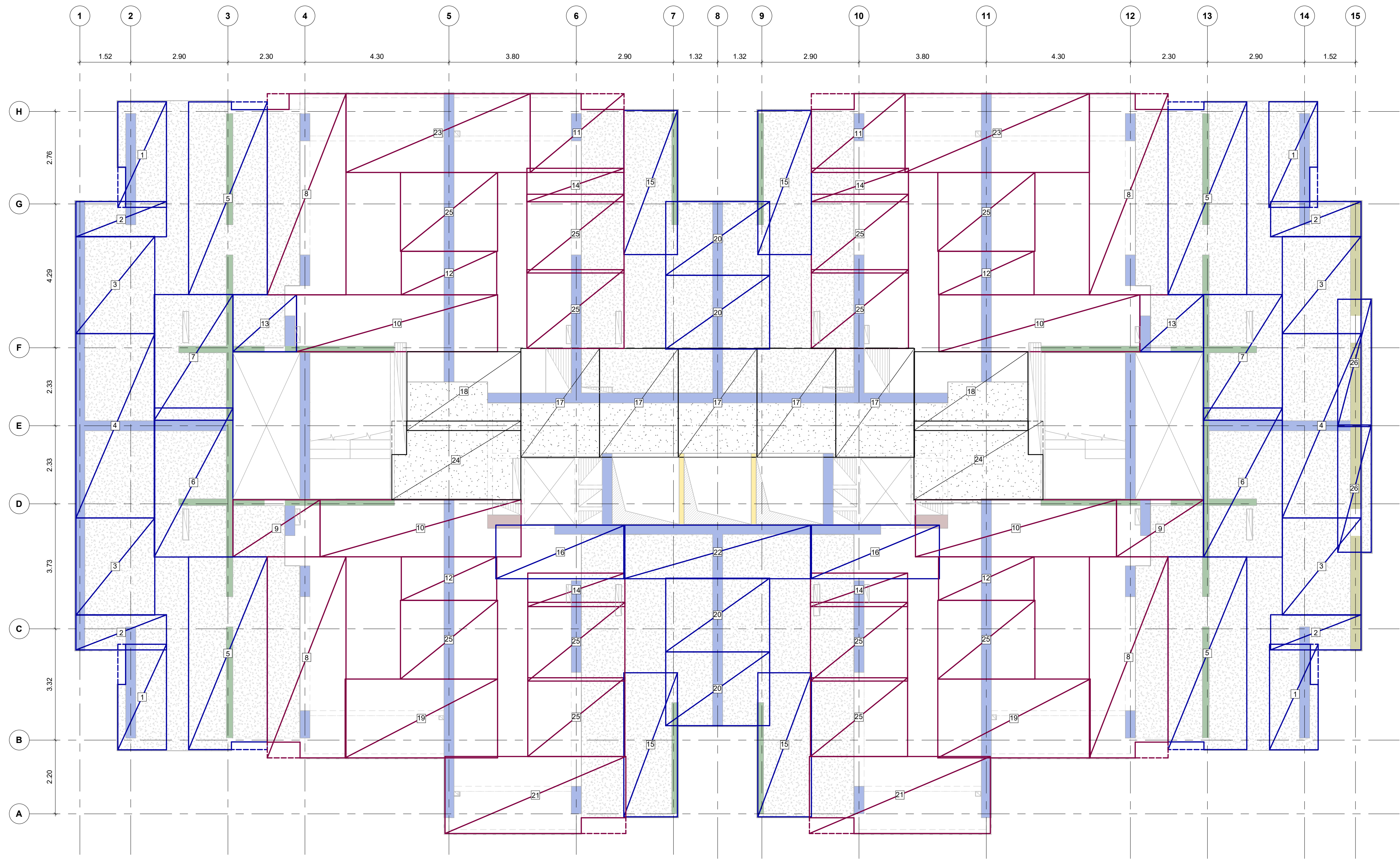
PLANTA DE REFUERZO SUPERIOR PISO TIPO 3 ( PISO 23 A PISO 28 ) Escala 1 : 75
